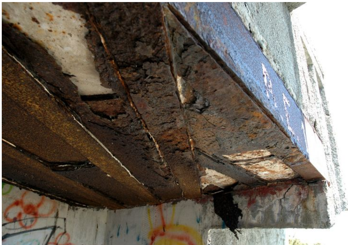
Vue du plafond de la chambre de tir du bunker - casemate de type 671 sud (état en 2005)
