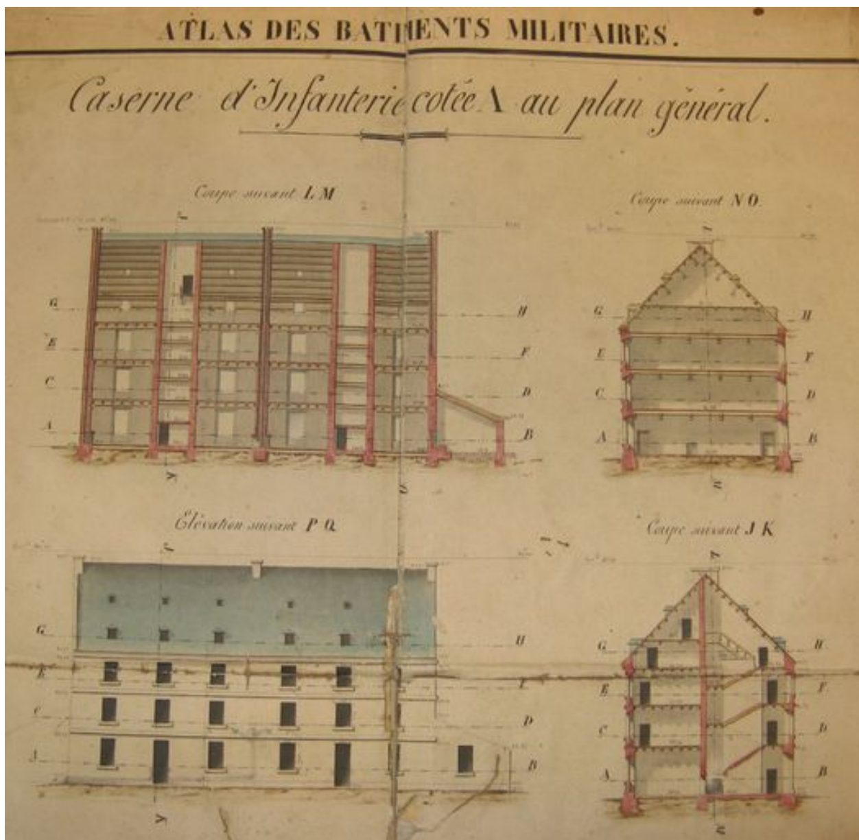
Plan de la caserne d'infanterie de Sourdís
