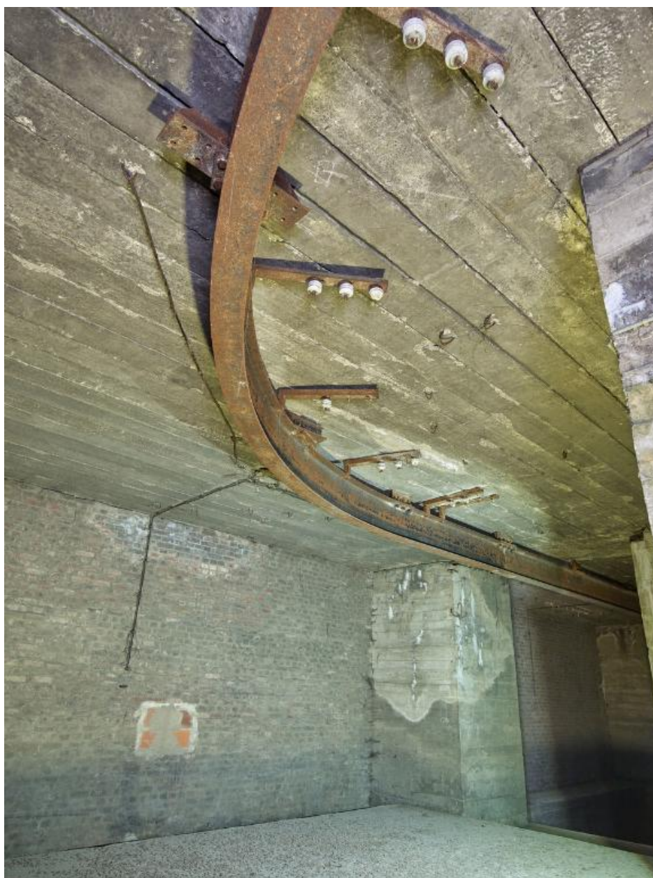
Vue du deuxième étage de l'extension sud : couloir d'accès aux trémies à charbon, monorail avec son système d'alimentation électrique triphasée. Au fond, les trois trémies
