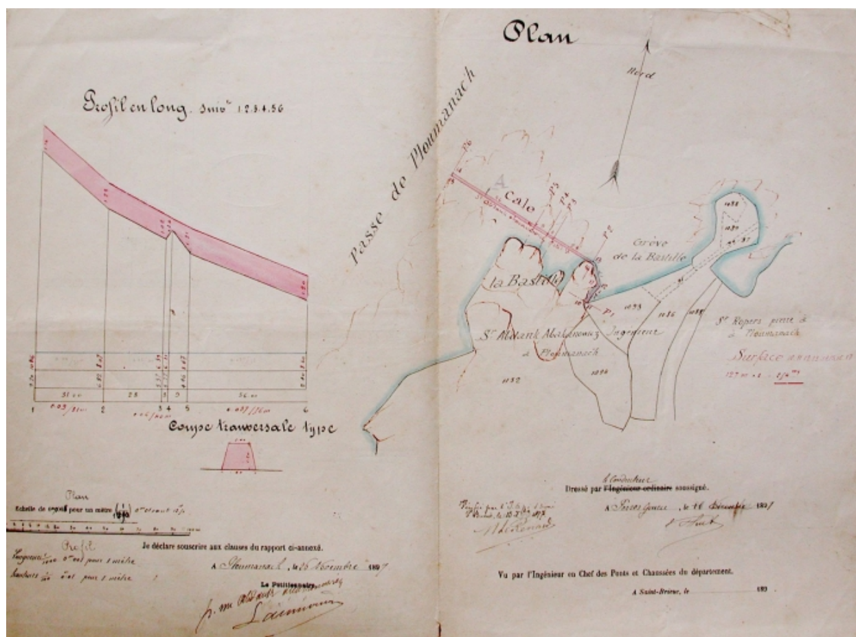
Plan : cale débarcadère du château de Costaeres, construite en 1896 (AD 22)
