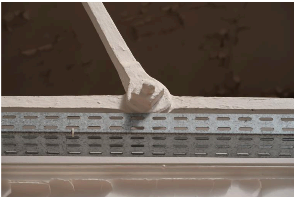
Vue intérieure : partie ouest, détail de l'un des tirants faisant "entrait" de la charpente métallique (état en 2022)
