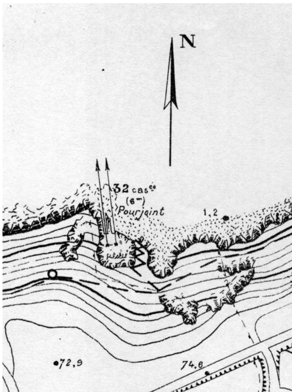
Extrait du plan de situation des batteries de Pourjoint et de la pointe des Espagnols : batterie casematée de 32 cm de Pourjoint, Atlas des batteries de côte : côte de Brest, 1913
