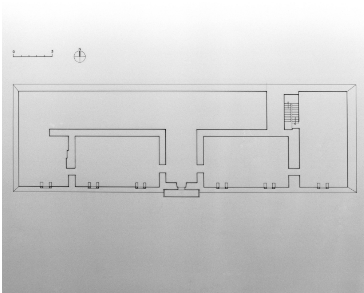
Plan des combles (relevé Atelier 3, Douarnenez, 1988)
