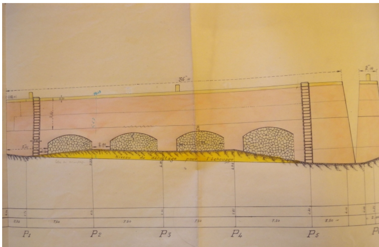
Plan du nouveau quai en béton sur voûtes, 1927 (AD 22)
