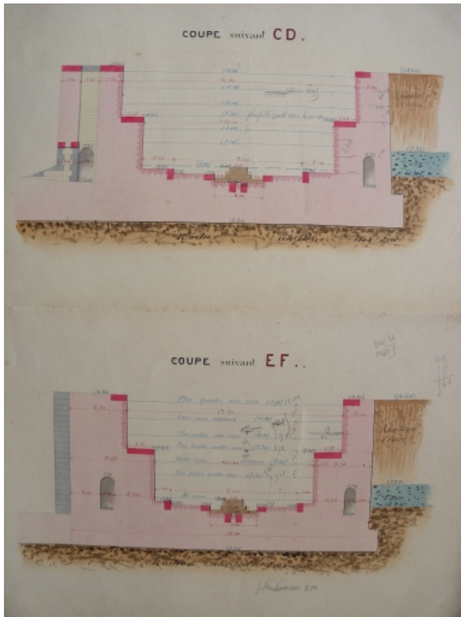
Plan : coupe en travers de la forme de radoub, 1883 (AD 22)
