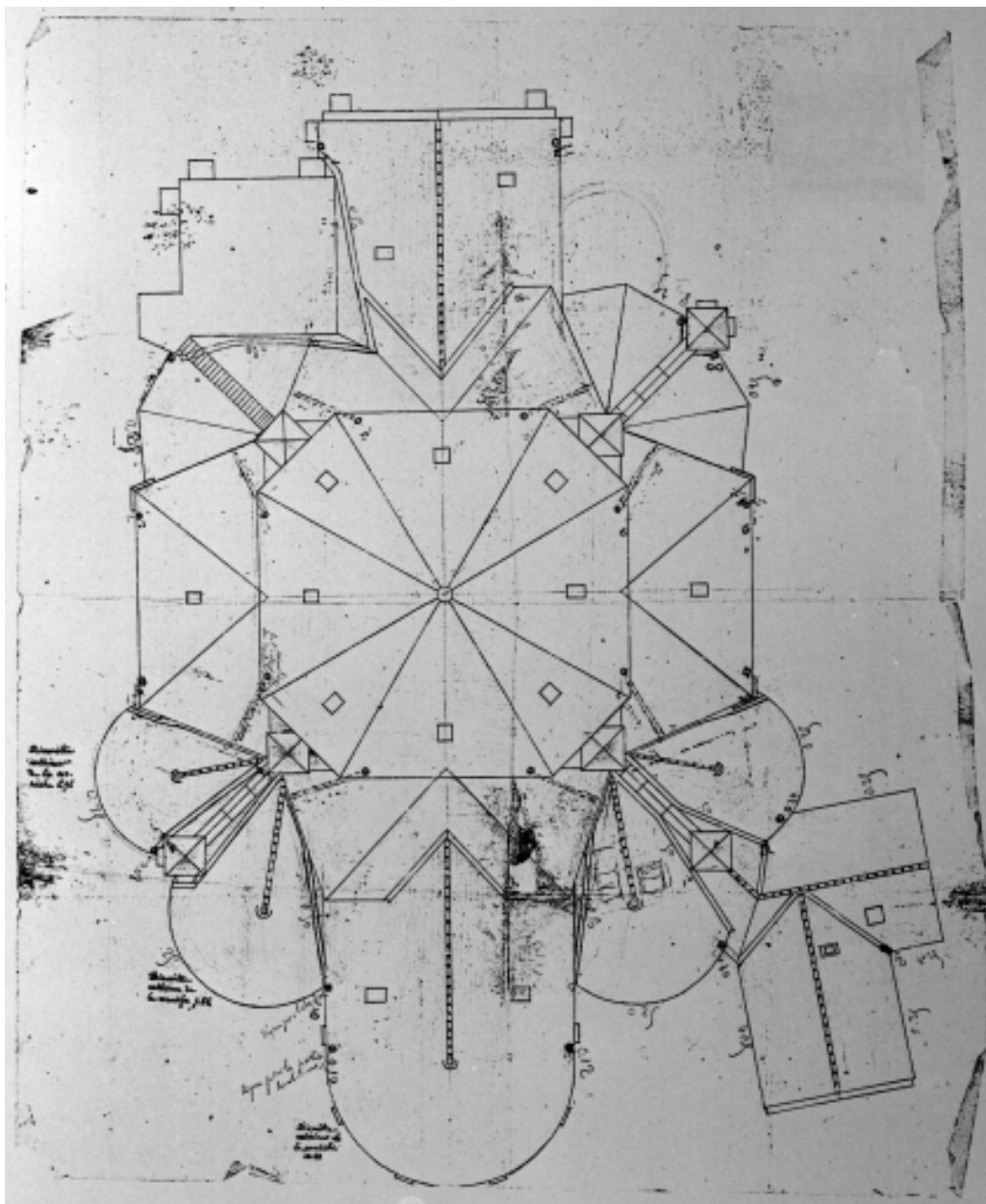
Plan dressé par Arthur Regnault à la fin du 19e siècle : plan des toits de l'église
