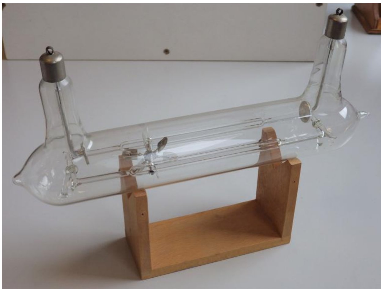
Tube de Crookes avec moulinet sur rails - Electricité dynamique (Non signé)
