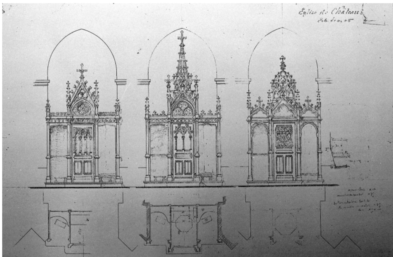
Elévations des confessionnaires.
