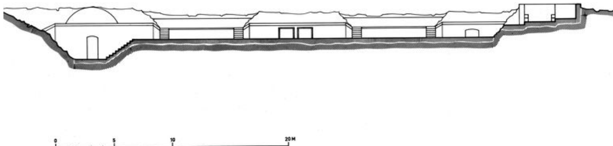
Elévation et coupe de la batterie de Tremet
