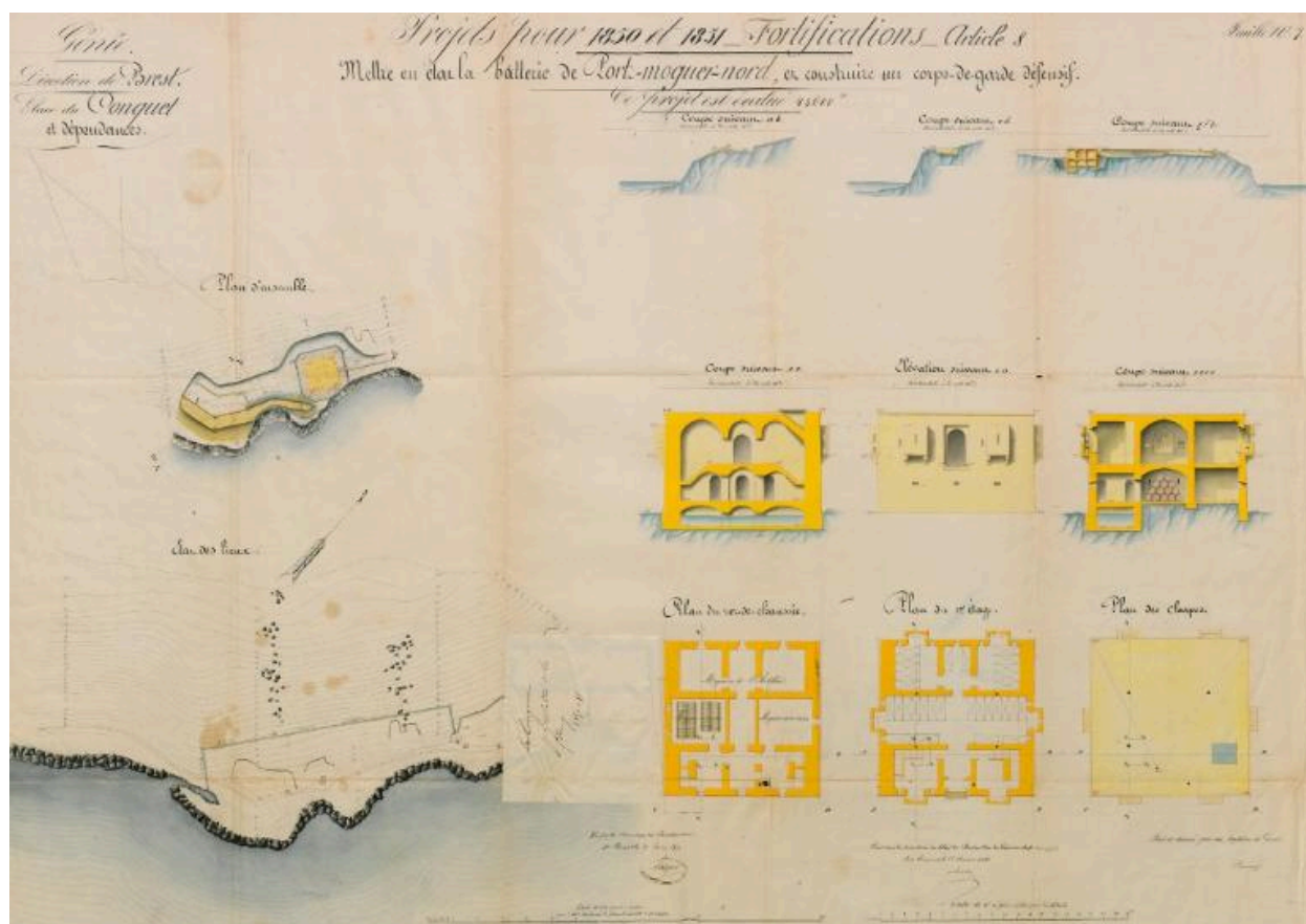
Plans, coupes et élévation de la tour-réduit de la batterie nord de Portzmoguer à Plouarzel, feuille de dessin des projets pour 1850-1851, 13 janvier 1850
