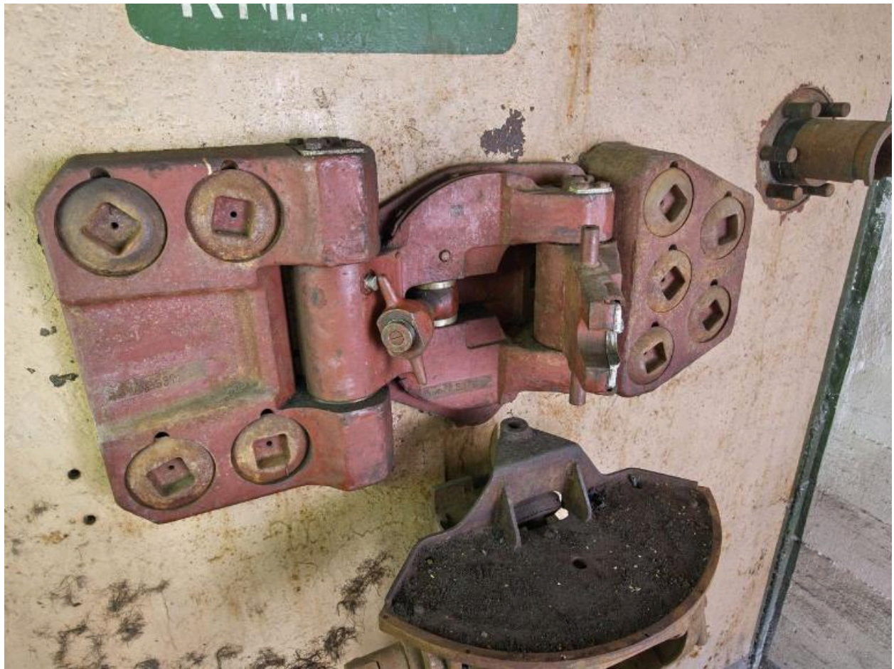
Vue du créneau blindé pour mitrailleuse avec support d'affût et affût
