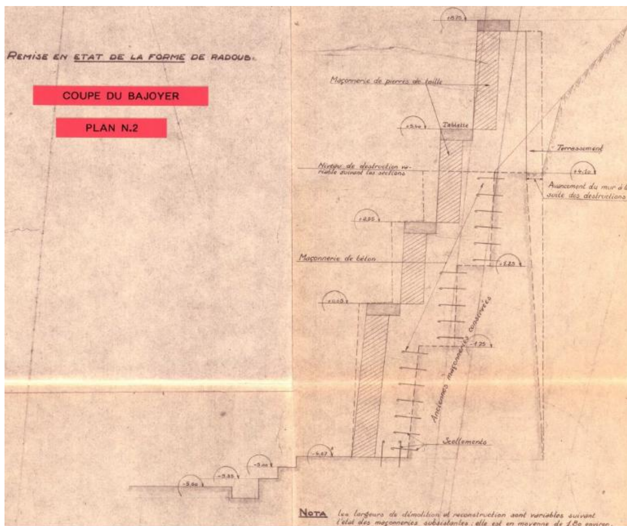
Remise en état de la forme de radoub, coupe bazoier (1948)
