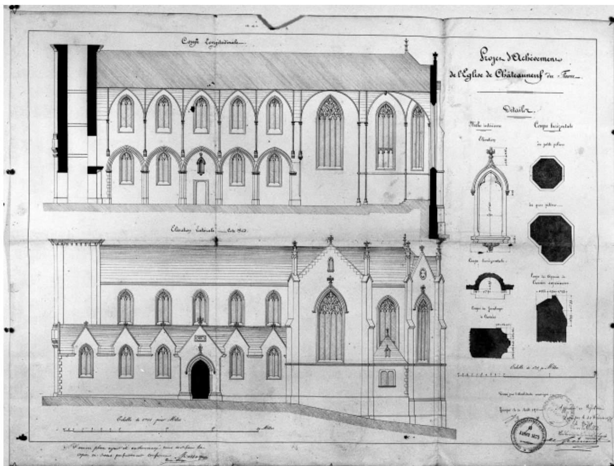
Châteauneuf-du-Faou, église paroissiale Saint-Julien et Notre-Dame : projet d'achèvement de l'église par Boyer, 1876 (coupe longitudinale, élévation sud Reproduction A.D. Finistère, IV, 307 de 1970)
