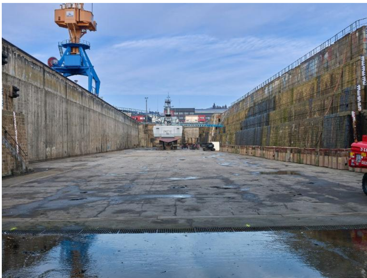
Radier et bajoyers de la forme 1
