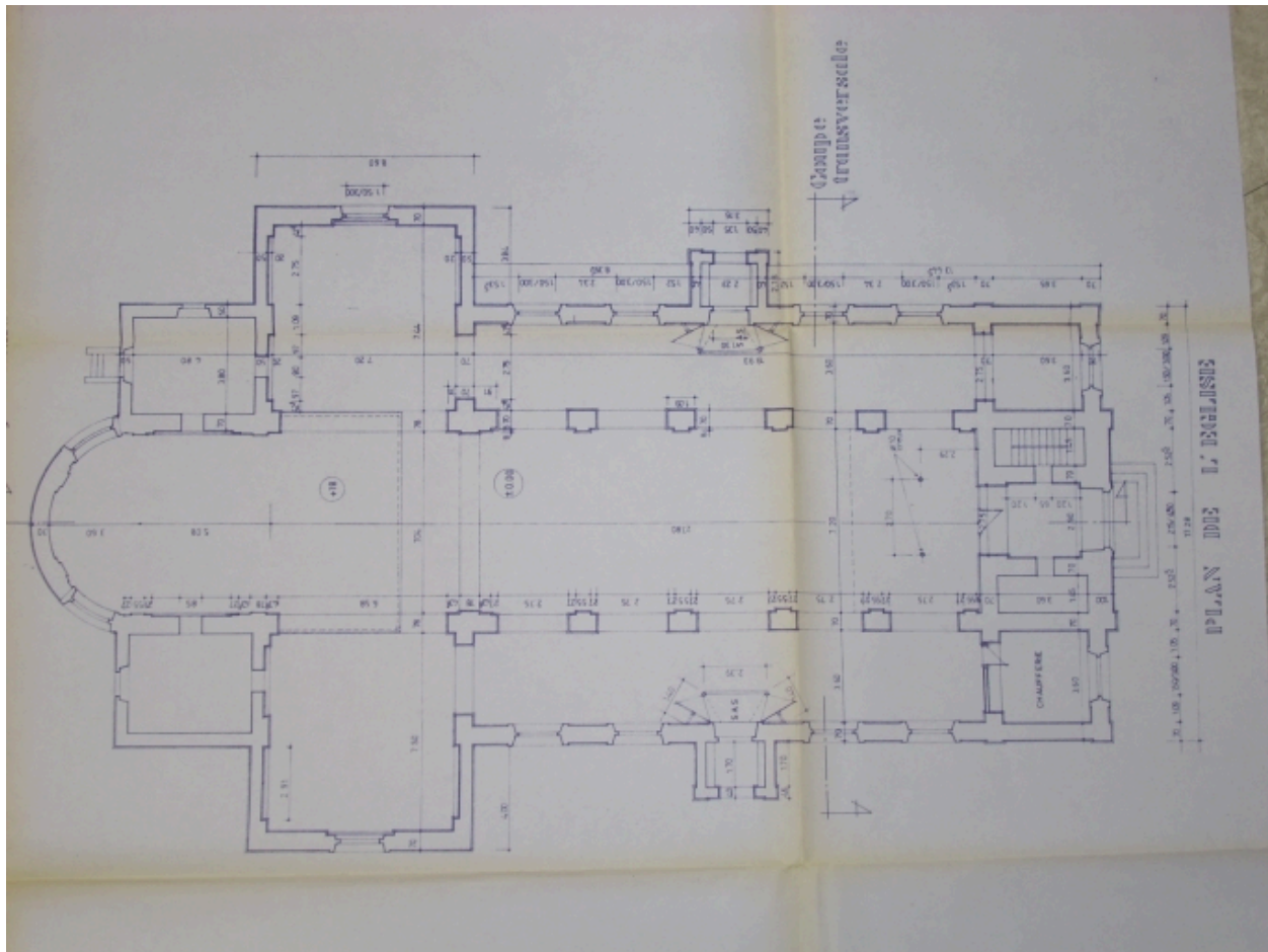
Plonéour-Lanvern, église paroissiale Saint-Eneour : plan au sol
