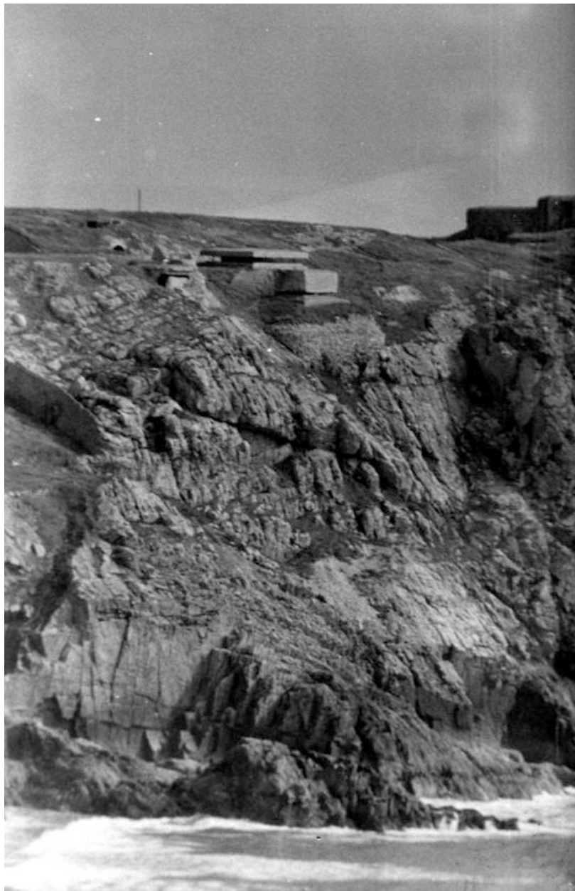
Vue de la batterie de Kerbonn en 1969 : bunker - poste de direction de tir de type M162a
