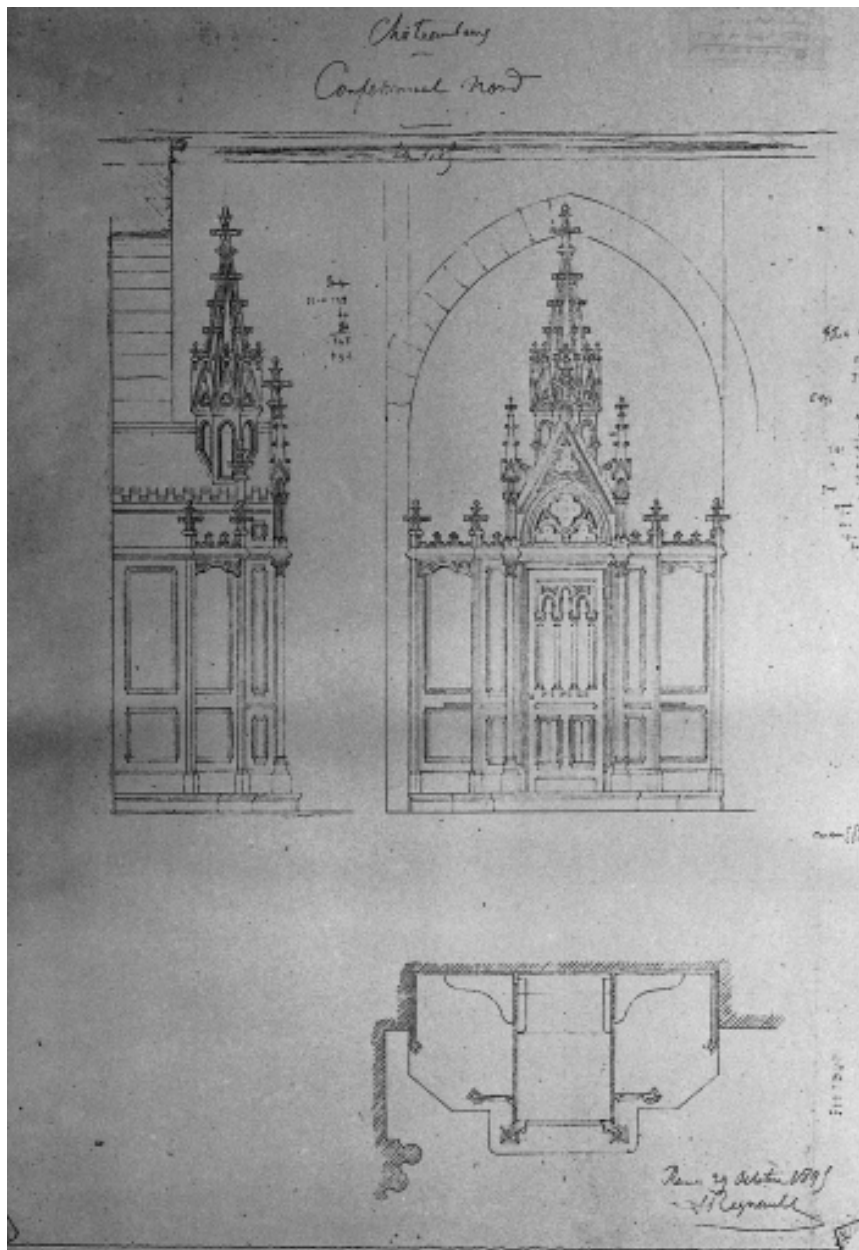
Confessionnal Nord : plan et élévation de face et de côté.
