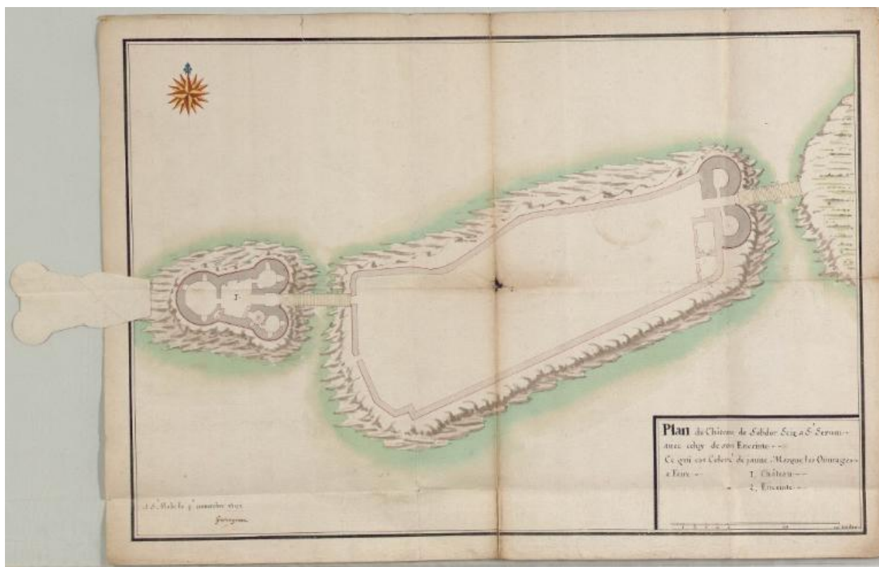
Plan du rez-de-chaussée de la Tour Solidor et de son ouvrage avancé par l'ingénieur Garengneau, 4 novembre 1691
