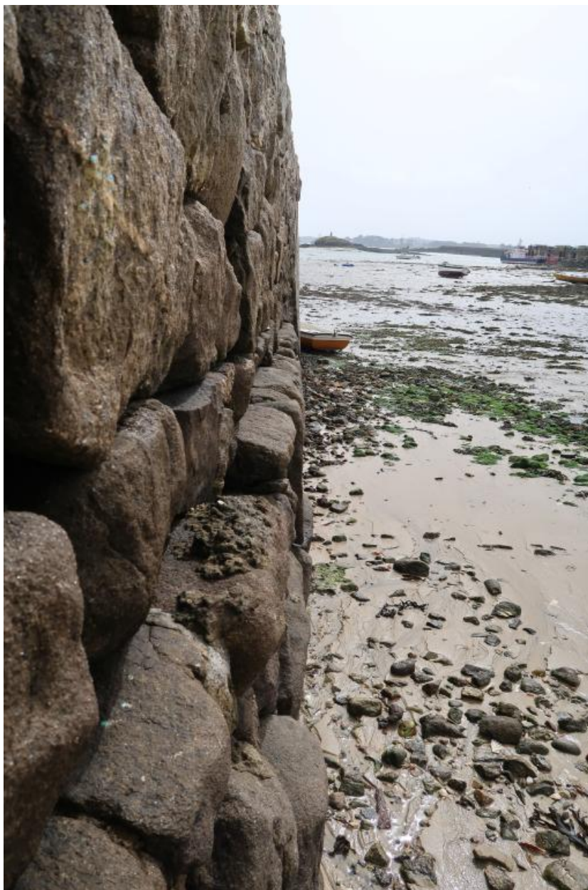
Cale de Porz Kernog, détail maçonnerie, côté est
