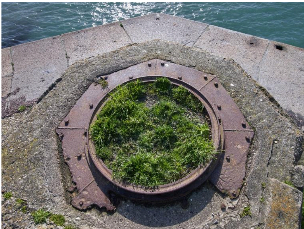
Vue de détail : chemin de roulement de la tourelle de char de combat
