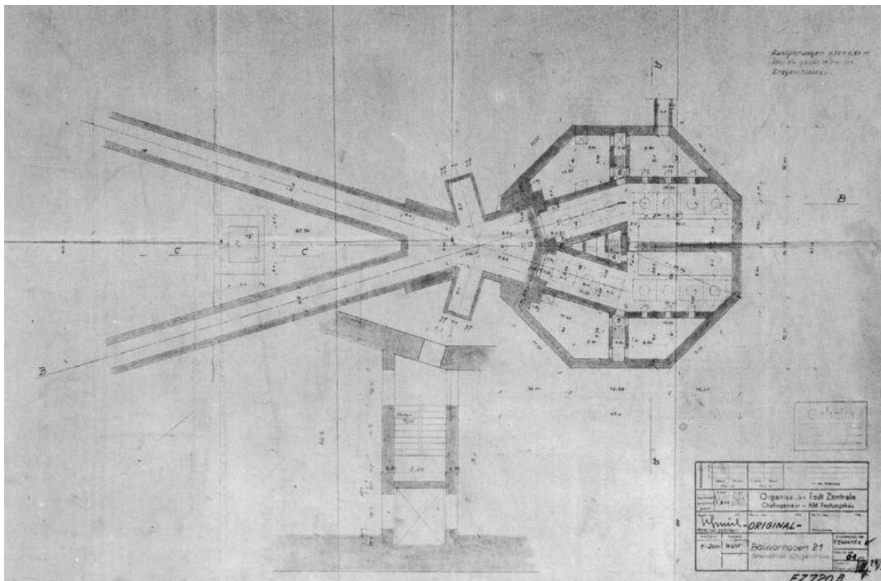
Plan du rez-de-chaussée de la base de V2 de Wizernes, Plan EZ 720 B (Bundesmilitärarchiv)
