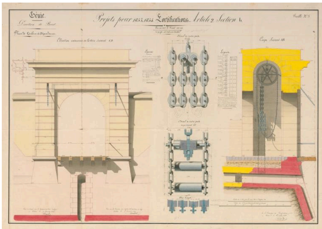
Place de Quéléren et dépendances, projets pour 1853-1854 : élévation et coupe de la porte avec pont-levis à contrepoids du fort de Quéléren, 22 décembre 1852
