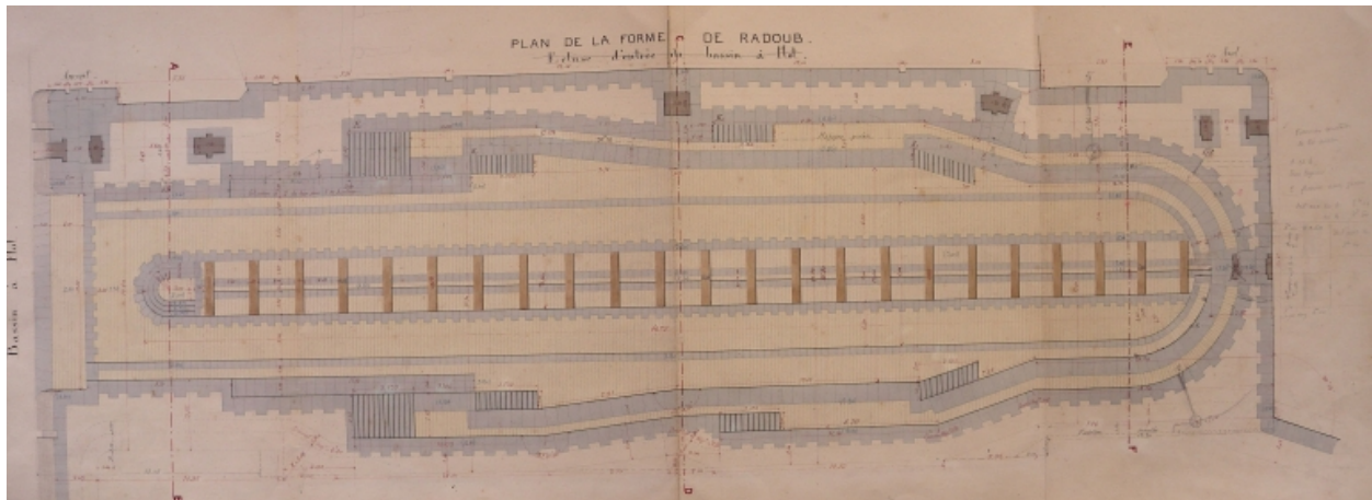
Plan de la forme de radoub, 1883 (AD 22)
