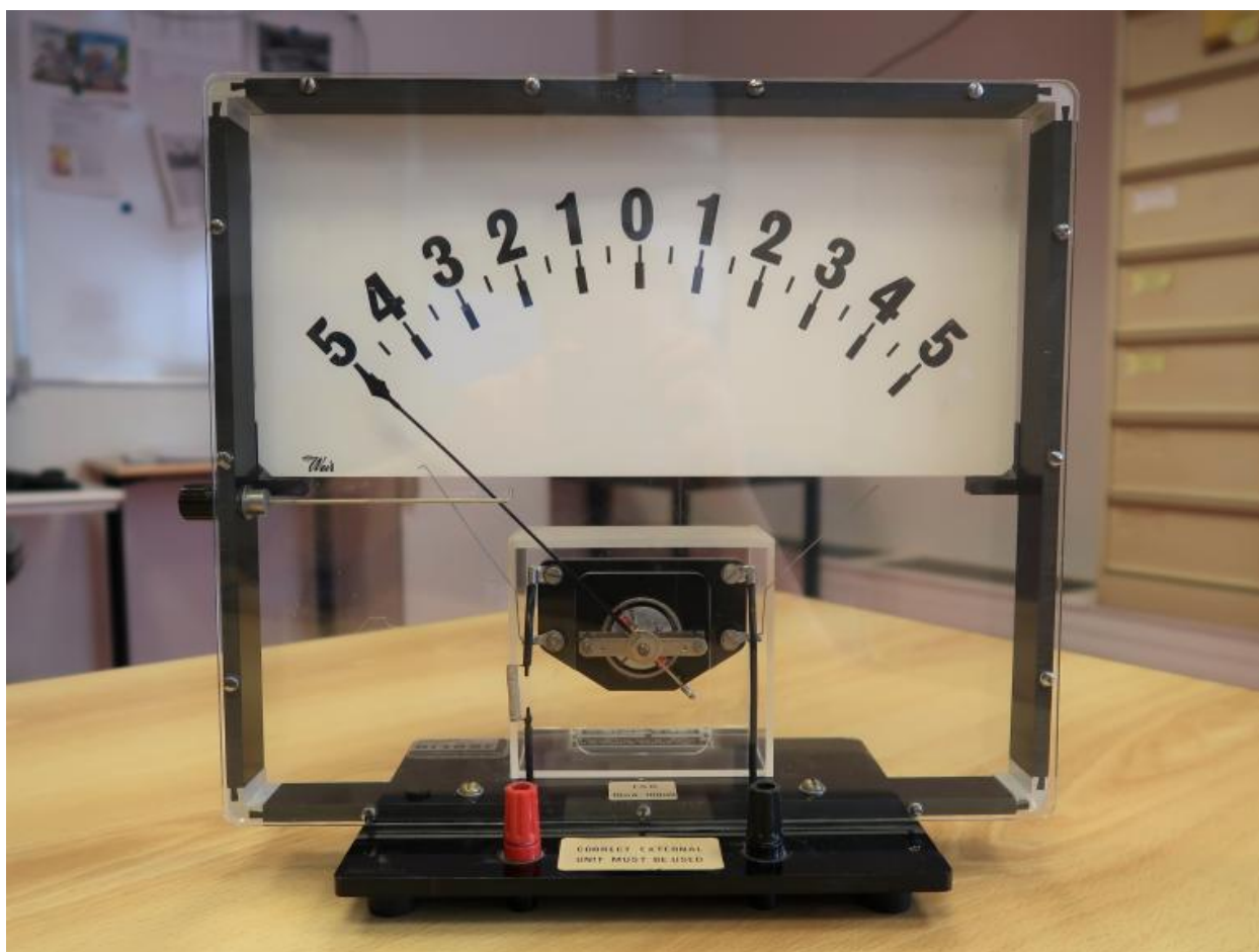
Galvanomètre - Electricité dynamique (Weir, distribué par Jeulin)
