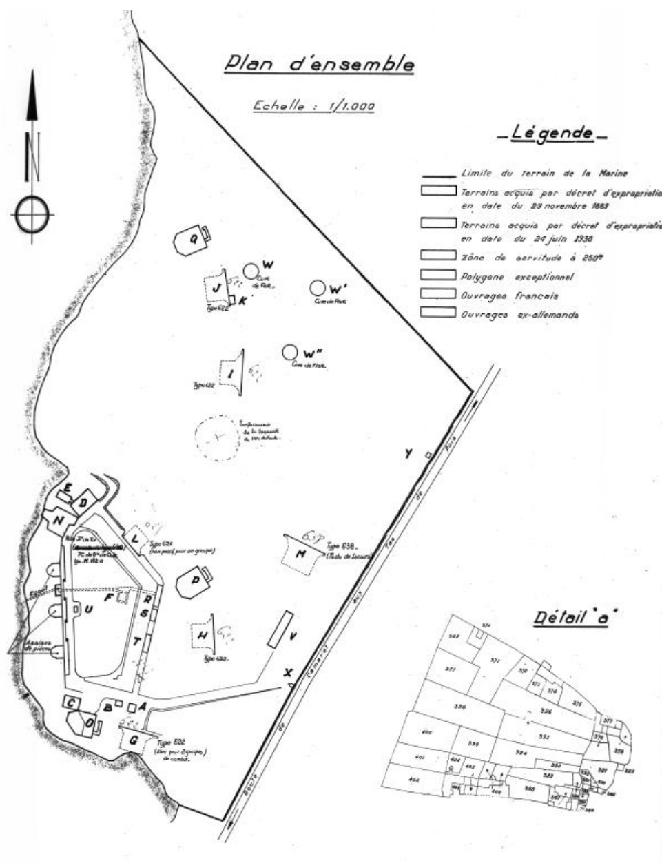
Plan d'ensemble de la batterie de Kerbonn (ouvrages français et ex-allemands)
