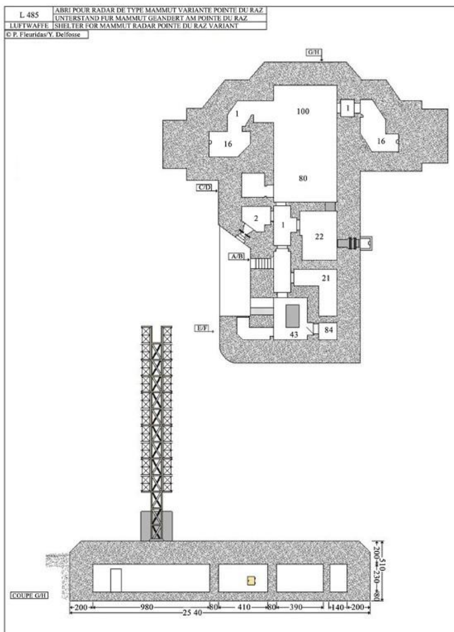
Plan et coupe du bunker de type L 485 pour radar Mammut (dessin : Patrick Fleuridas, Yves Delfosse)
