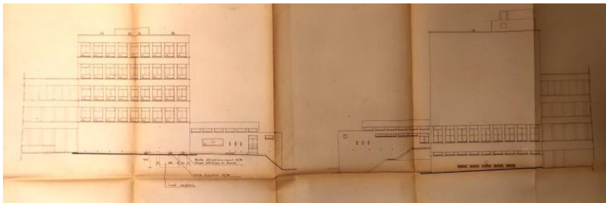
Internat - Bâtiment A. Façades nord et sud. Yves Moignet, architecte, 1960.
