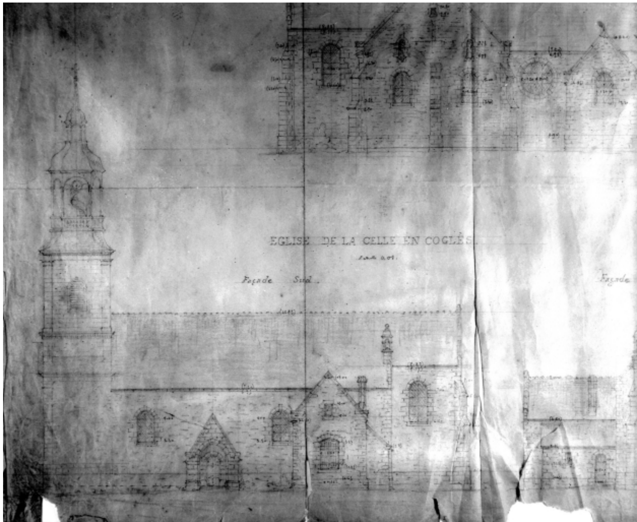
Élévation de la façade Sud de l'église.
