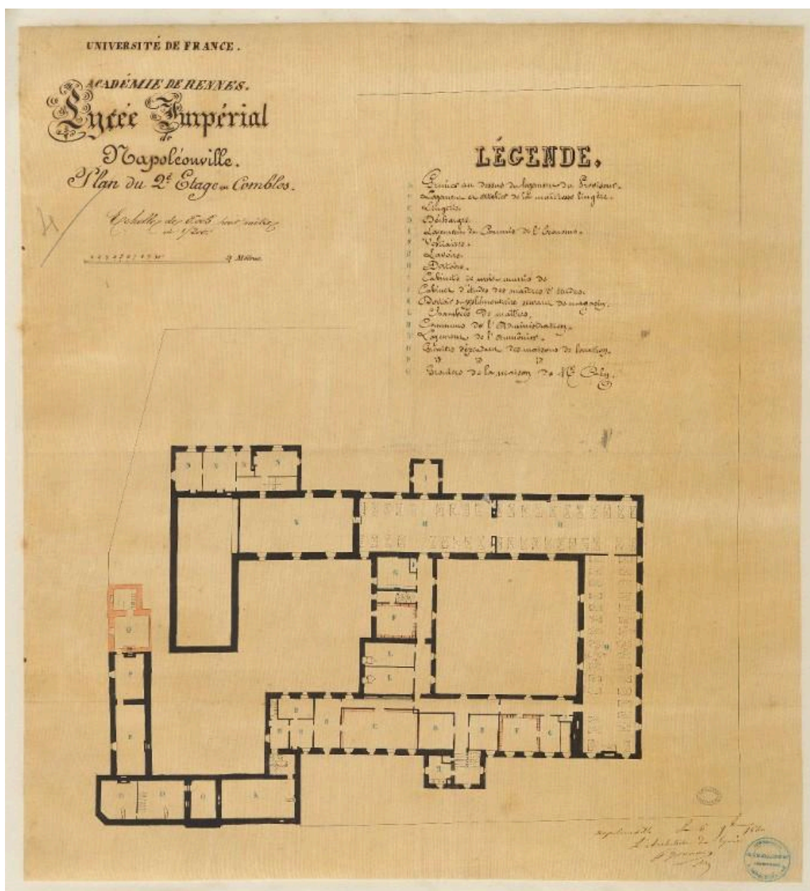
Lycée impérial de Napoléonville. Plan du 2e étage ou combles. 1842.
