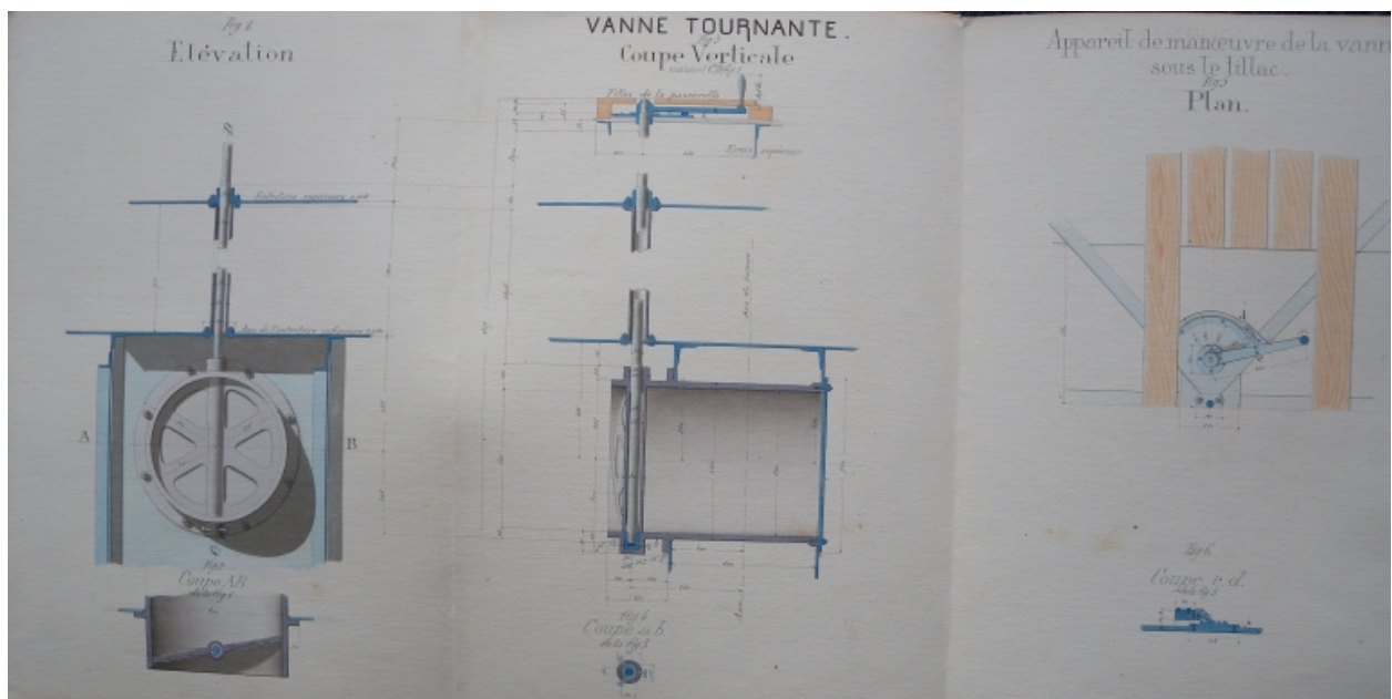
Plan : vue des vannes tournantes du bateau-porte en projet, 1886 (AD 22)
