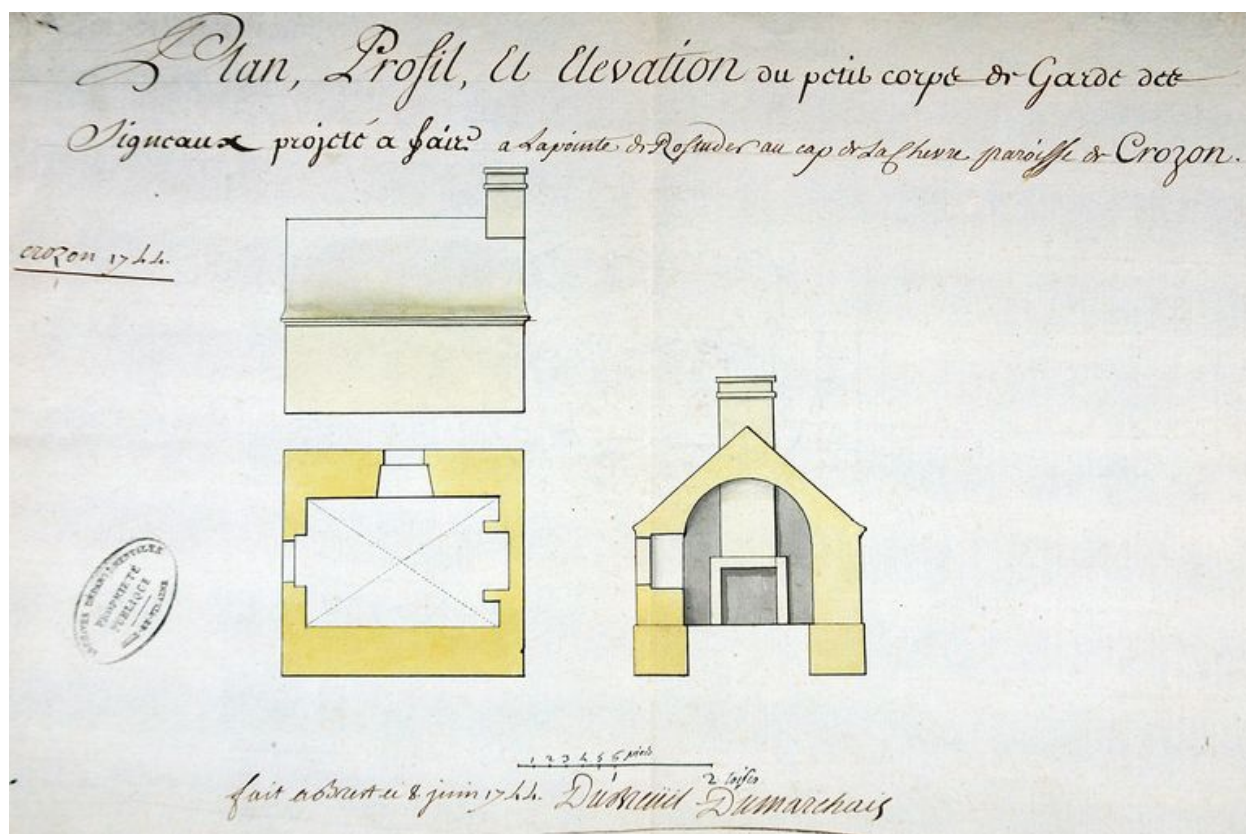
Elévation, plan et profil d'un petit corps de garde des signaux projeté à faire à la pointe de Rostuder au cap de la Chèvre dans la paroisse de Crozon, fait à Brest le 8 juin 1744 par Dubreuil Dumarchais
