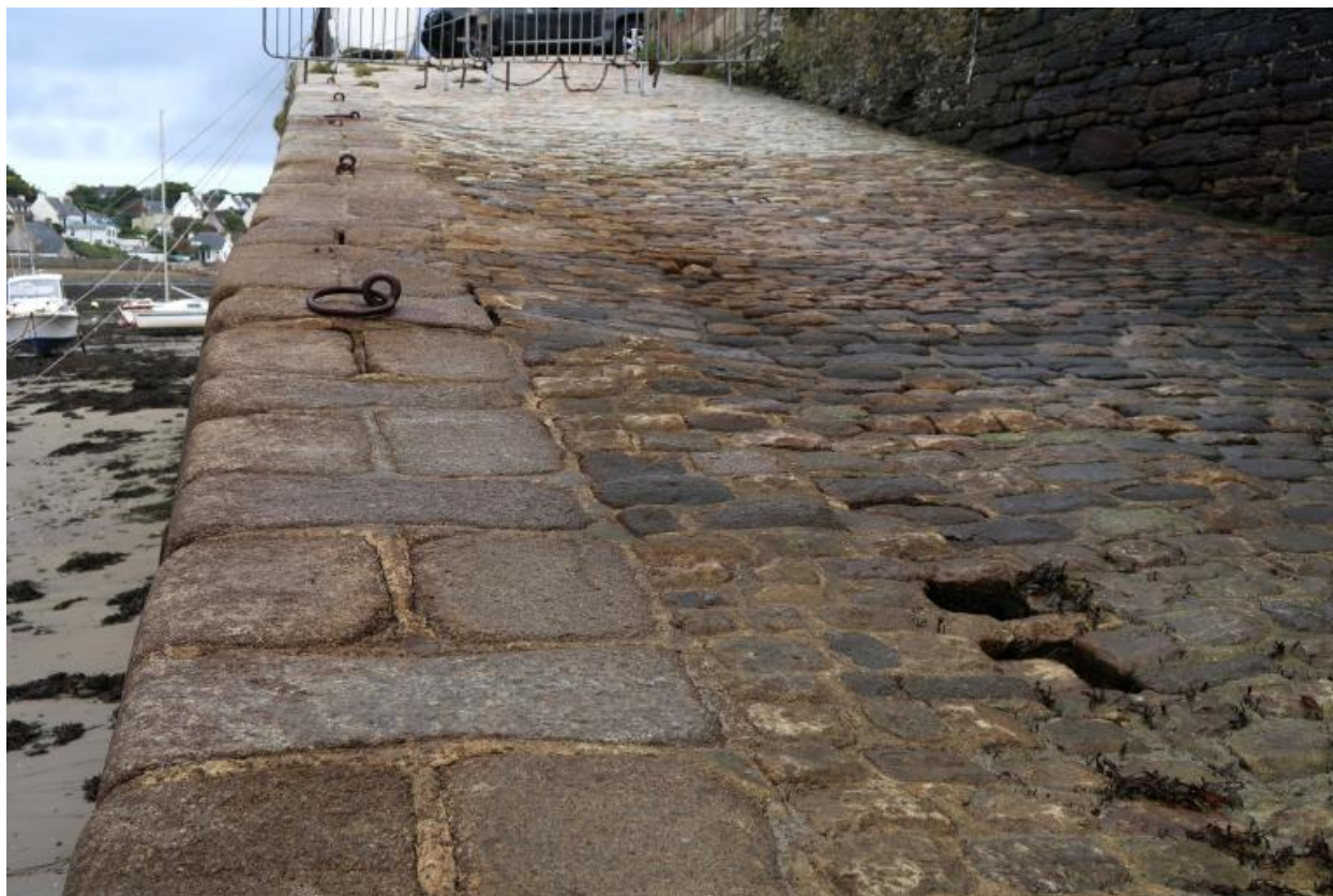
Cale Est : maçonnerie, organeaux. Platelage présentant des faiblesses
