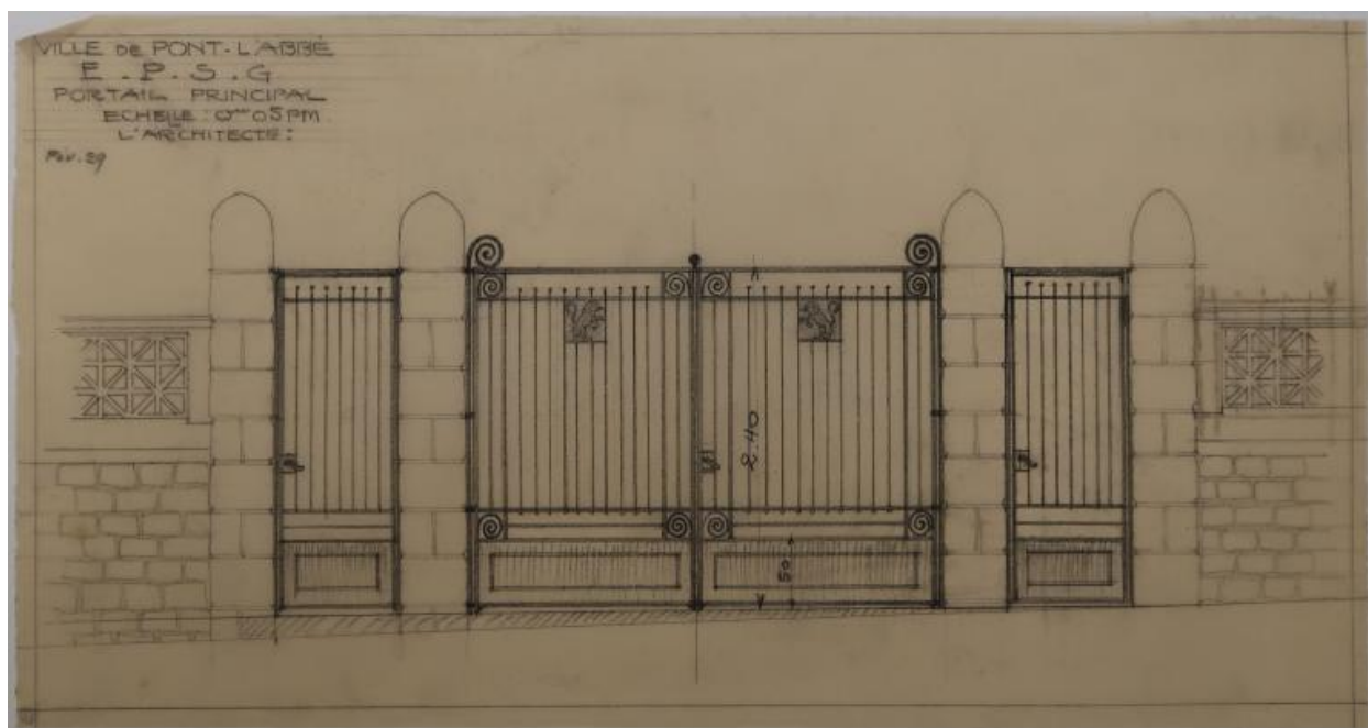
Portail principal. G-R. Lefort, architecte, février 1929.
