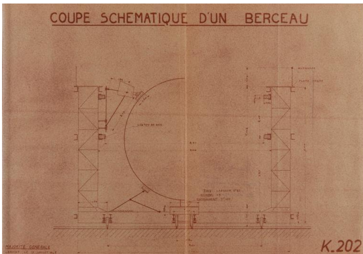
Coupe schématique du berceau du slipway, plan K n° 202, 17 juillet 1945 (Service Historique de la Défense de Lorient, Monographie de la base "Ingénieur Général Stoskopf", 1945-1946)
