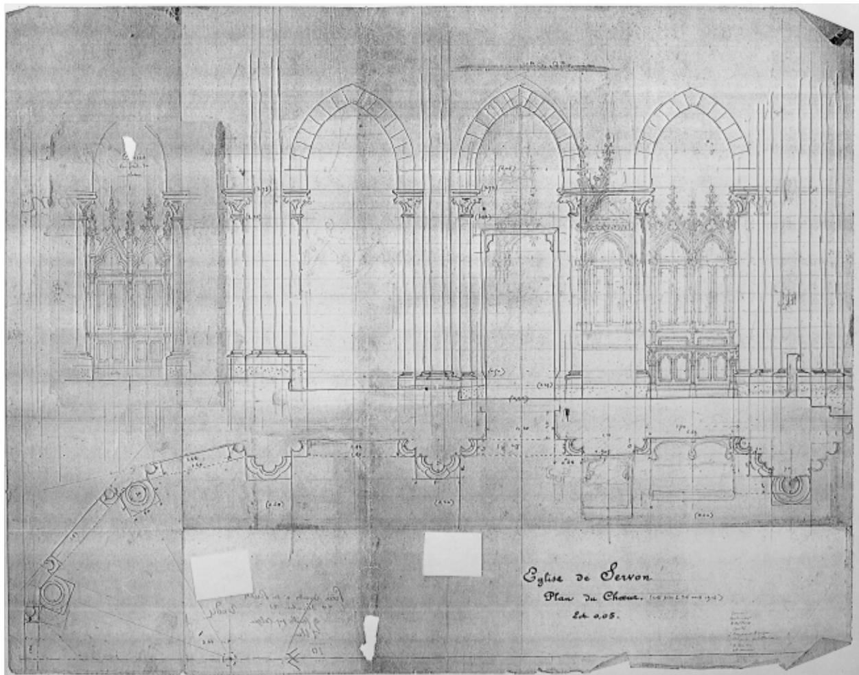
Plan du choeur, 1914, attribué à A. Regnault
