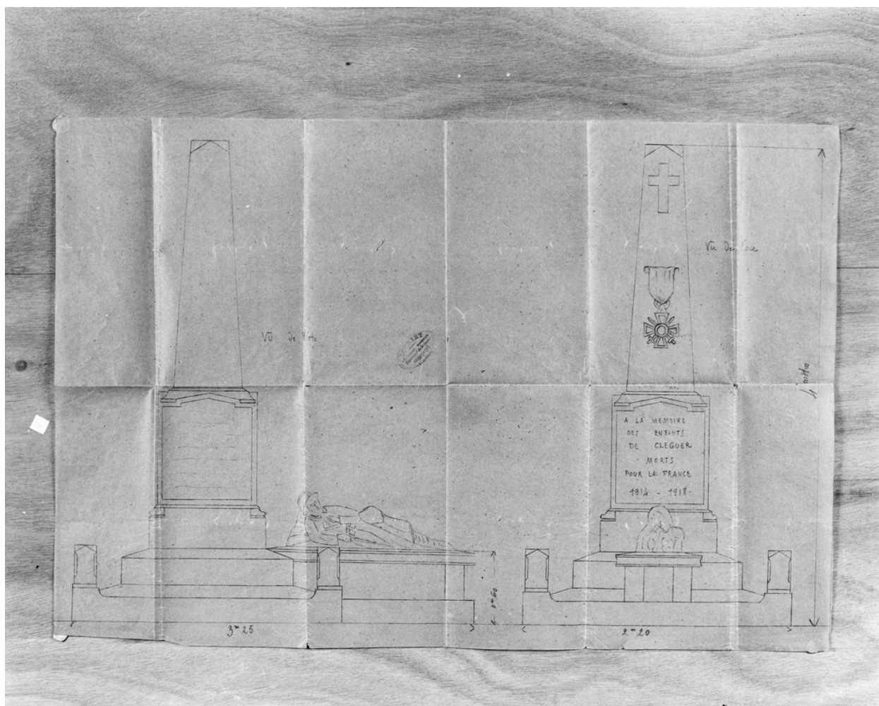
Plan de face et de côté du monument aux morts (1914-1918),
