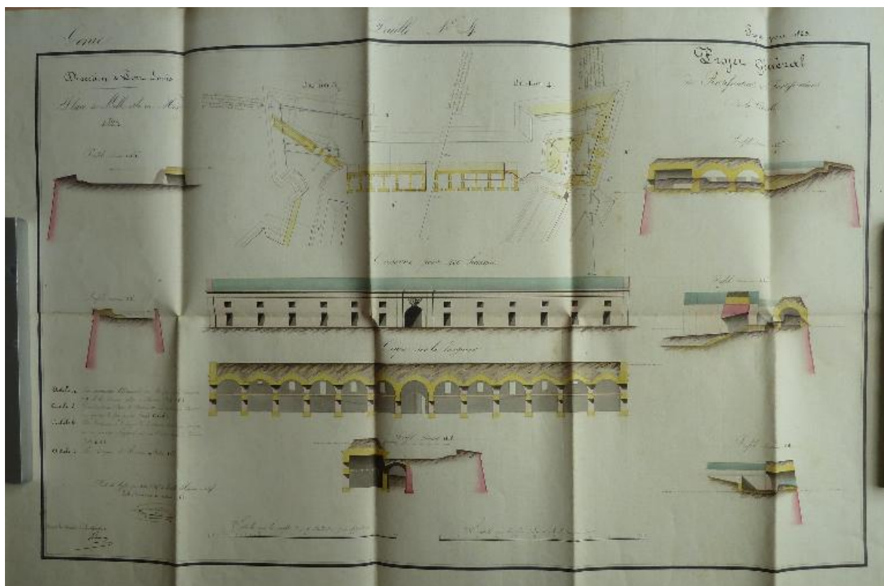
1 VH 287. Place de Belle-isle-en-Mer, feuille n° 4 des projets pour 1823, projet général de rectification des fortifications de la citadelle, 15 novembre 1822.
