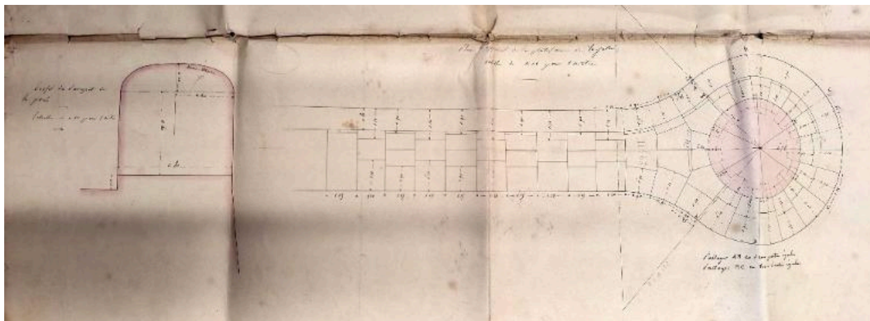
Plan et profil de la jetée du phare de la pointe de l'Aigle (7 novembre 1855)
