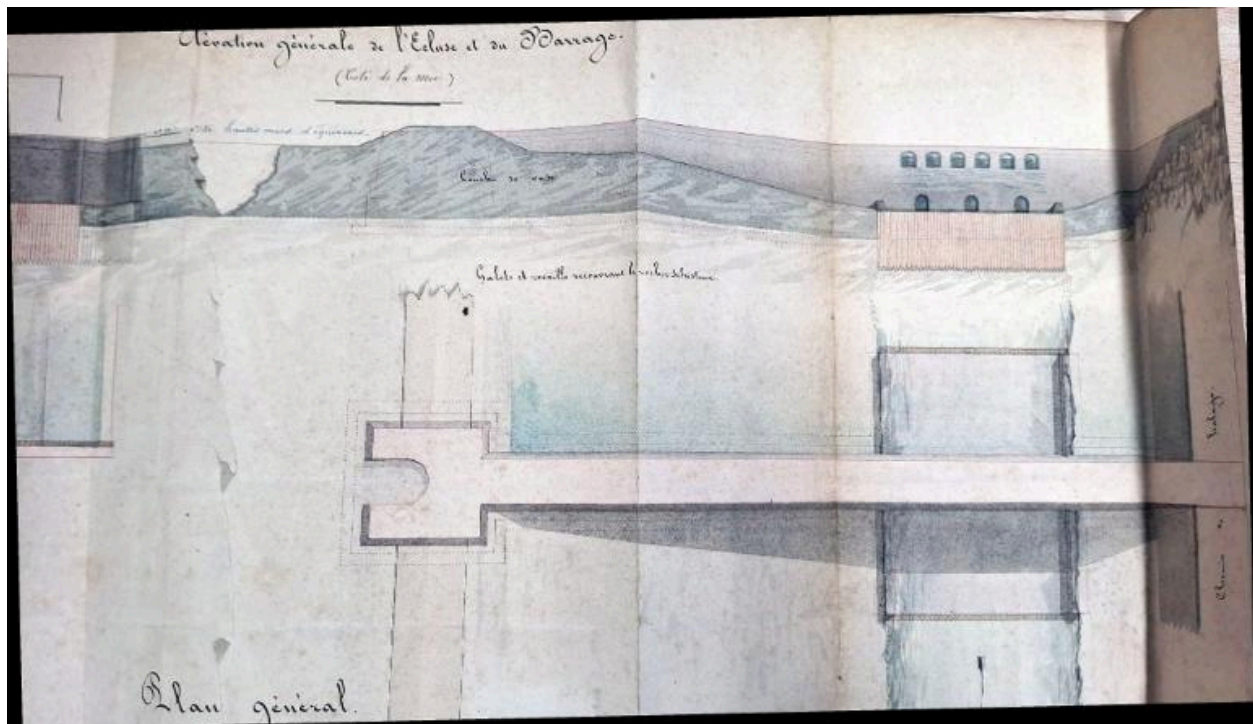
Avant-projet d'établissement de port à flot par le barrage de la vallée, 1er octobre 1839
