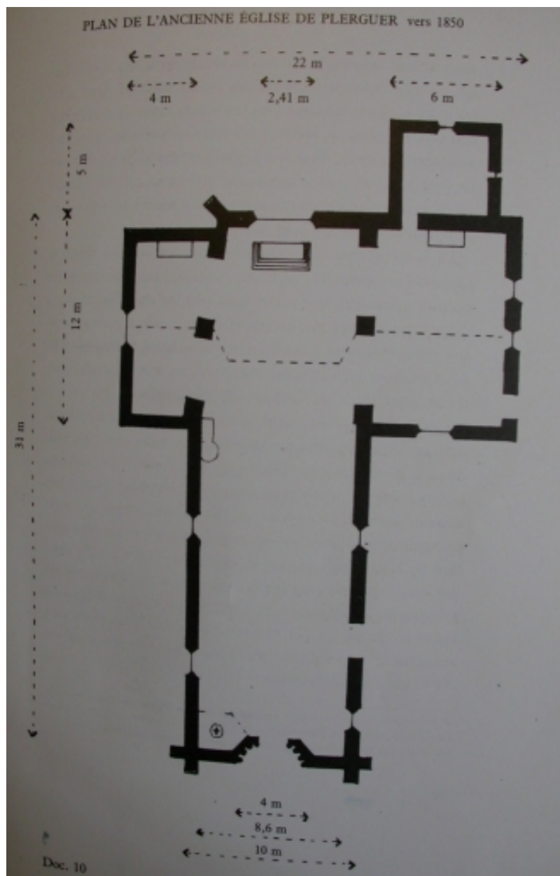
Plan de l'ancienne église
