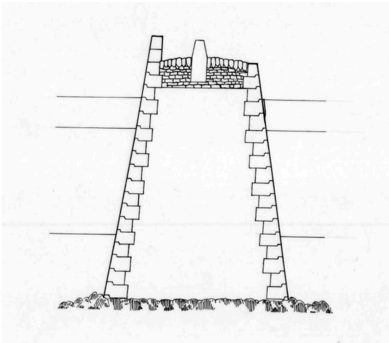
Coupe du môle (dessin JC. Fichou)
