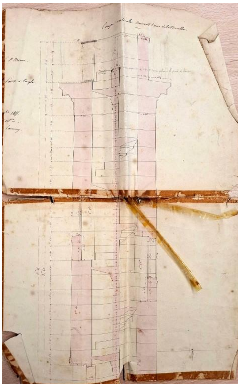
Coupe verticale du phare de la pointe de l'Aigle (18 novembre 1855)
