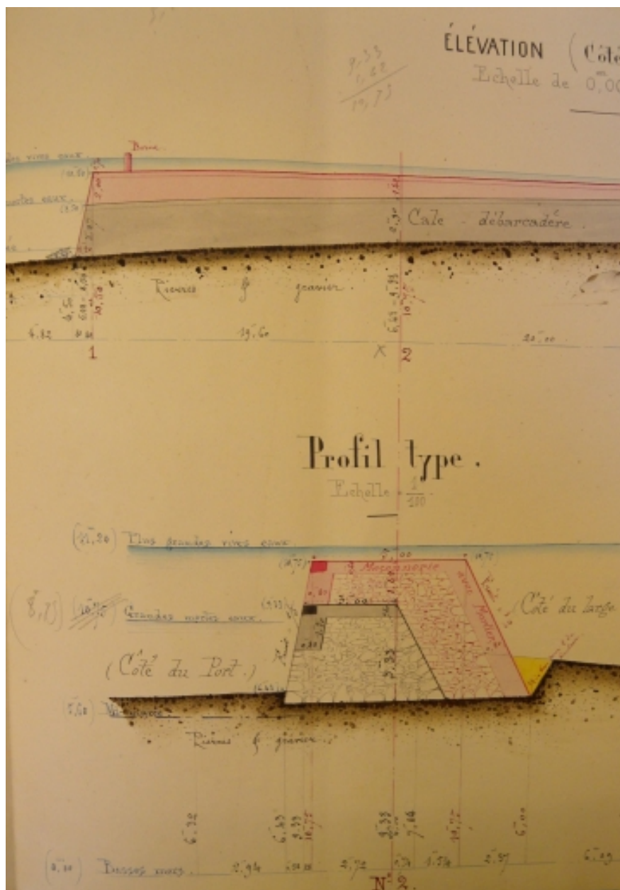
Profil type : avant-projet d'exhaussement de la cale, 1886 (AD 22)
