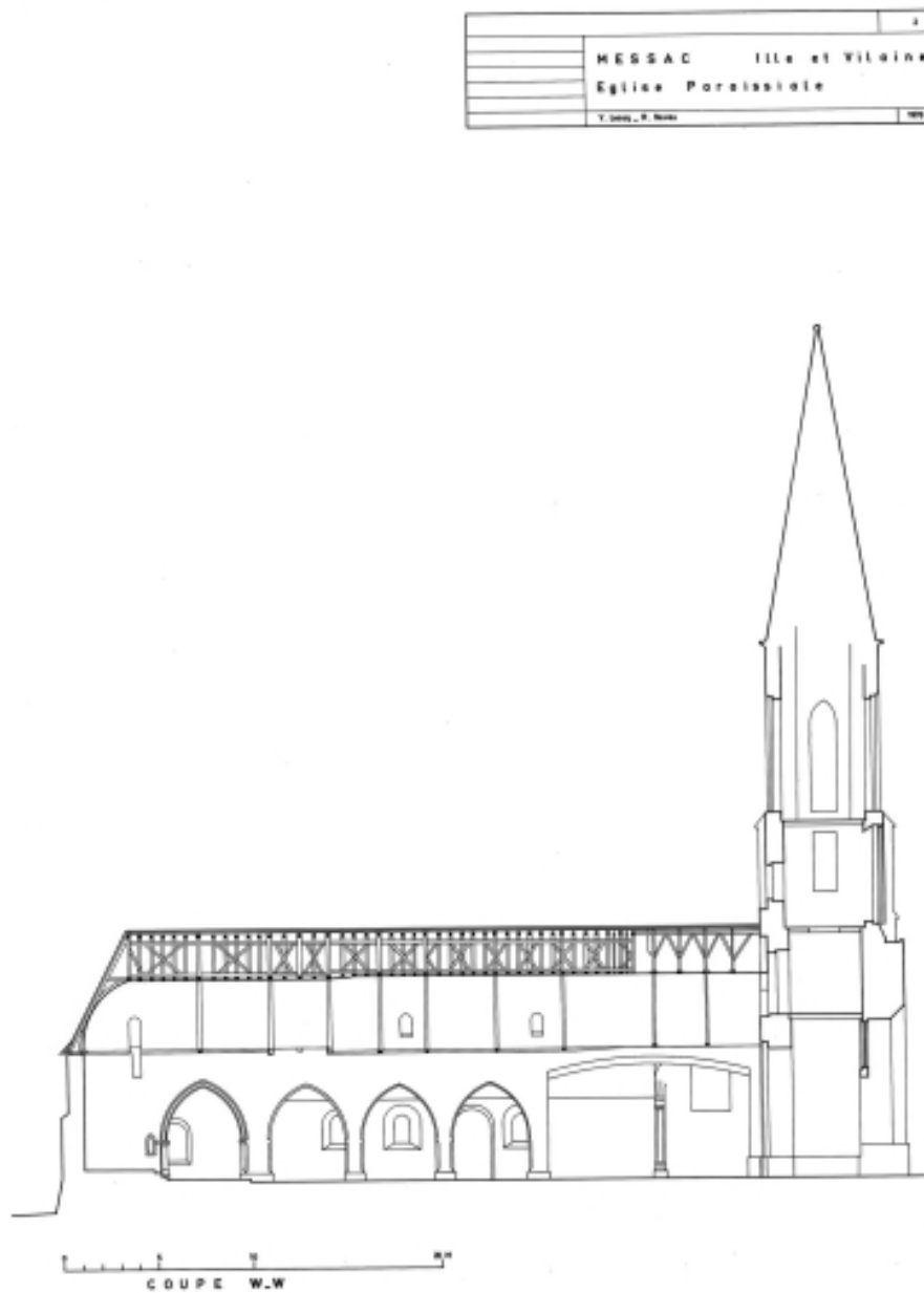
Coupe longitudinale Nord-Sud.
