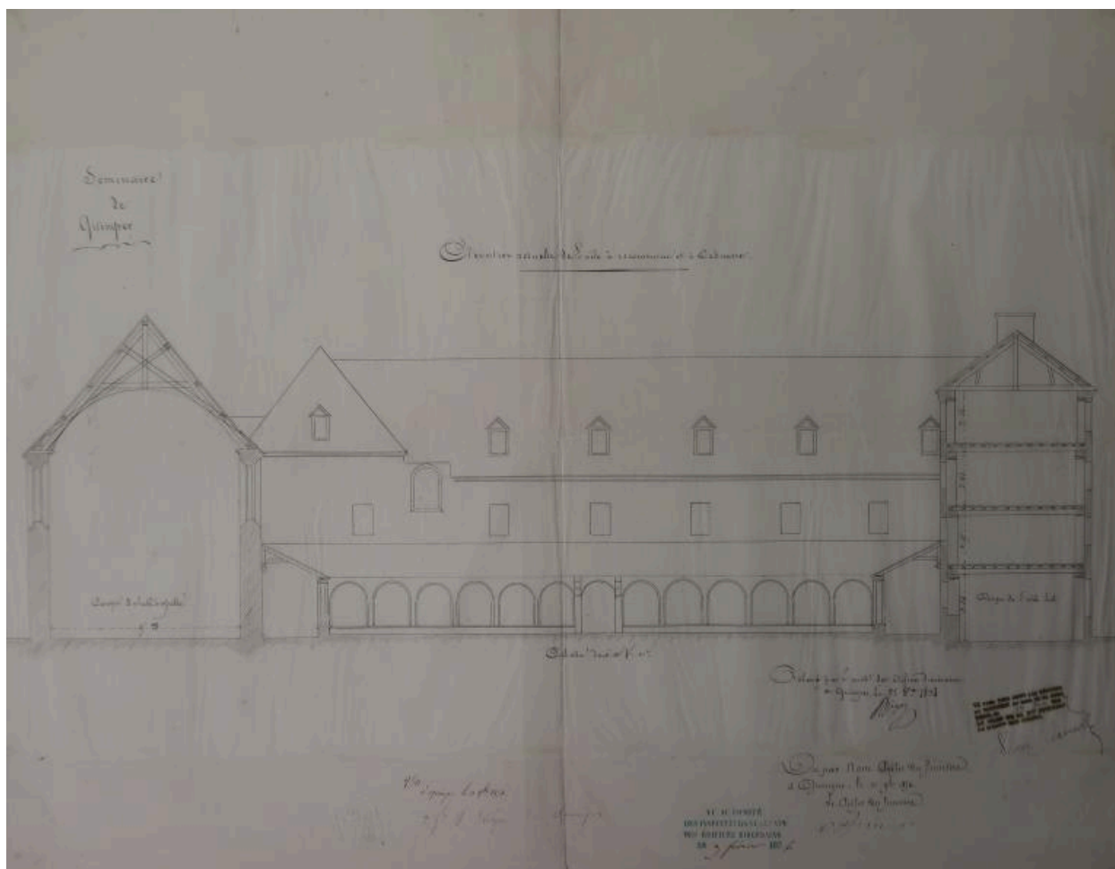
Élévation actuelle de l'aile à reconstruire et à exhausser (côté cour). Relevé réalisé par Joseph Bigot, architecte, 1854.
