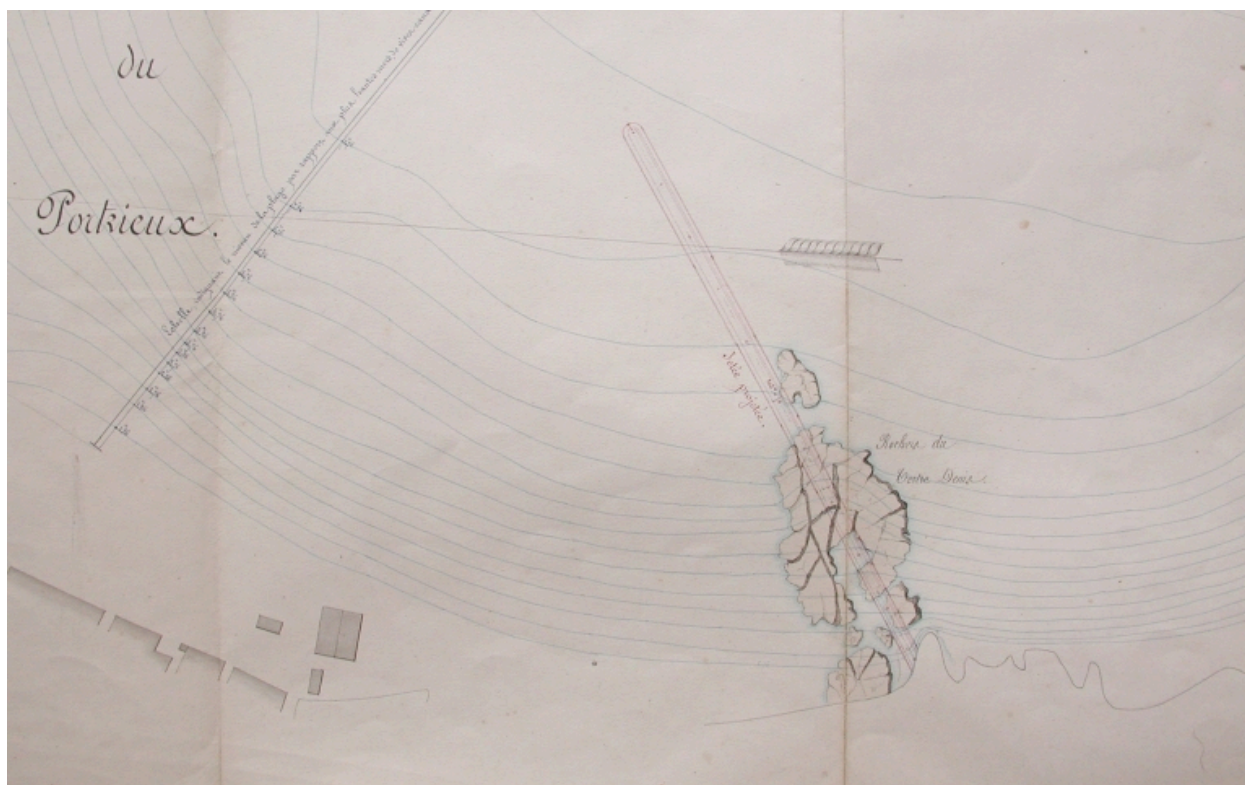
Plan : jetée projetée sur le rocher du Tertre Denis, 1854 (AD 22)
